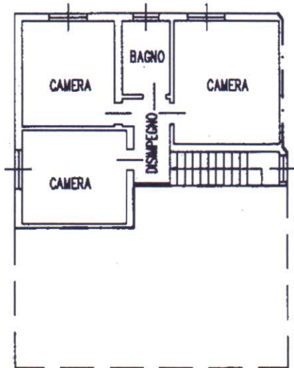
Sub 3 _ Pianta Piano Primo _ H=2.90
