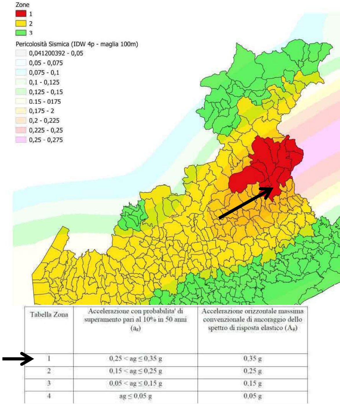
Fig. 6 – estratto della Zonizzazione Sismica di cui alla DRGV n. 244 del 09/03/2021 Classificazione sismica del Veneto Mappa di pericolosità sismica
