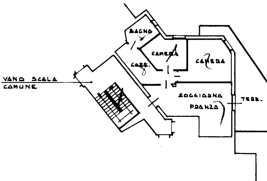
PIANO PRIMA H.2.80
